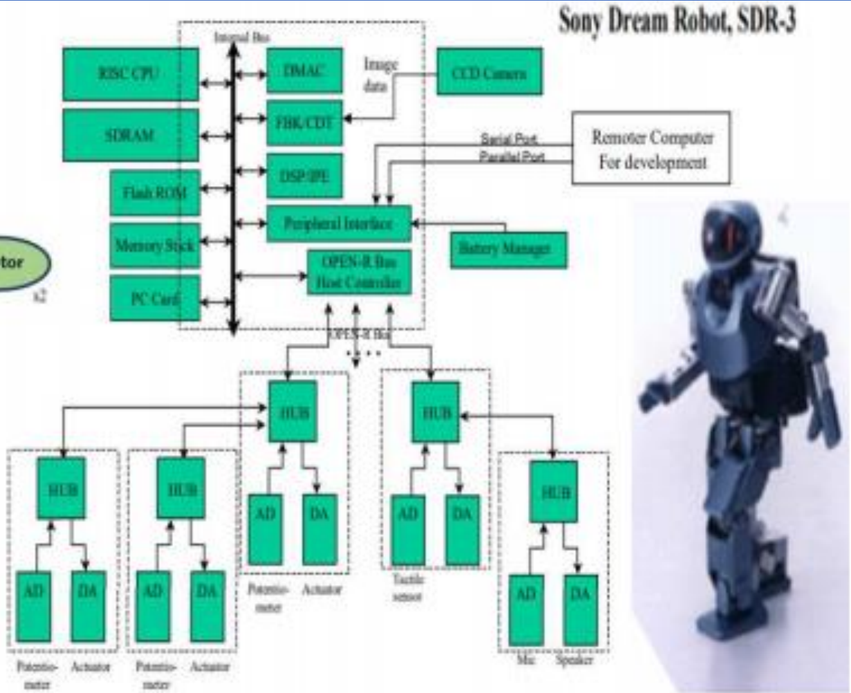
Sony Dream Robot AIBO ERS-210 and SDR-3.
