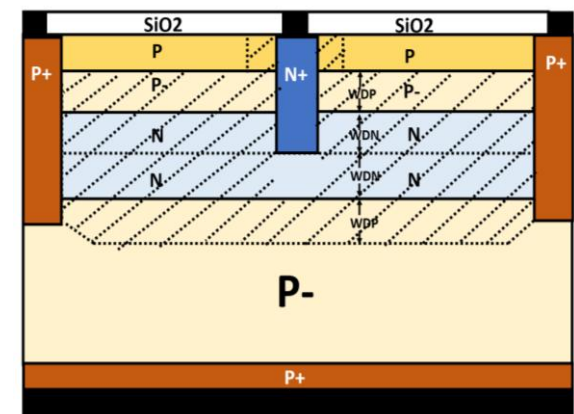
(D) Double P+PP-NP-P+接合型太陽電池 (Silicon Etching by KOH)
