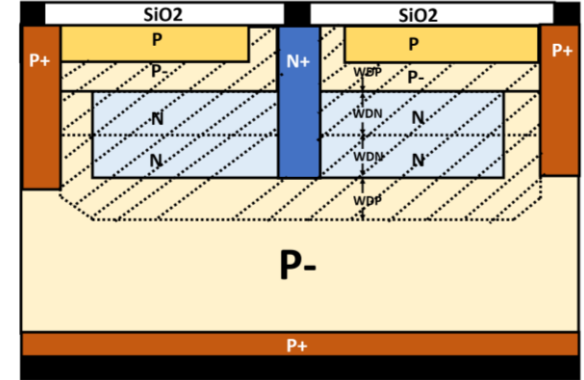
(D) Double P+PP-NP-P+接合型太陽電池
