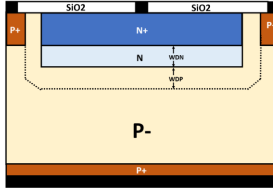
(B) Single N+NP-P+接合型太陽電池
