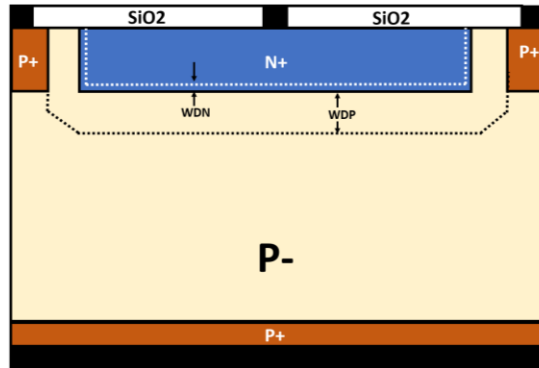
(A) 従来のSingle N+P-P+接合型太陽電池
