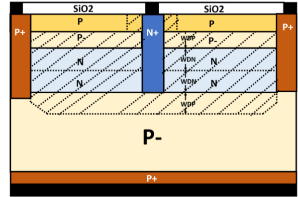
(C) Double P+PP-NP-P+接合型太陽電池
