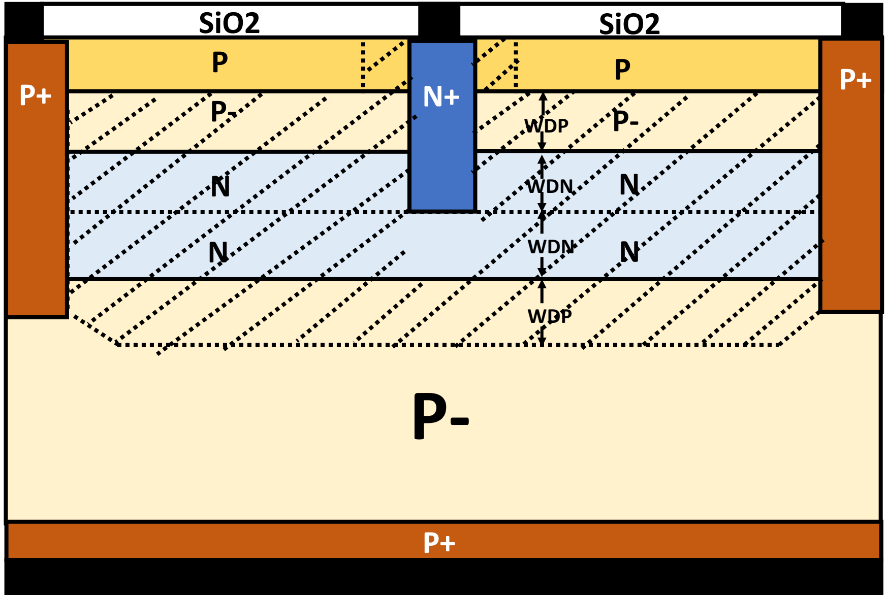
(C) Double P+PP-NP-P+接合型太陽電池
